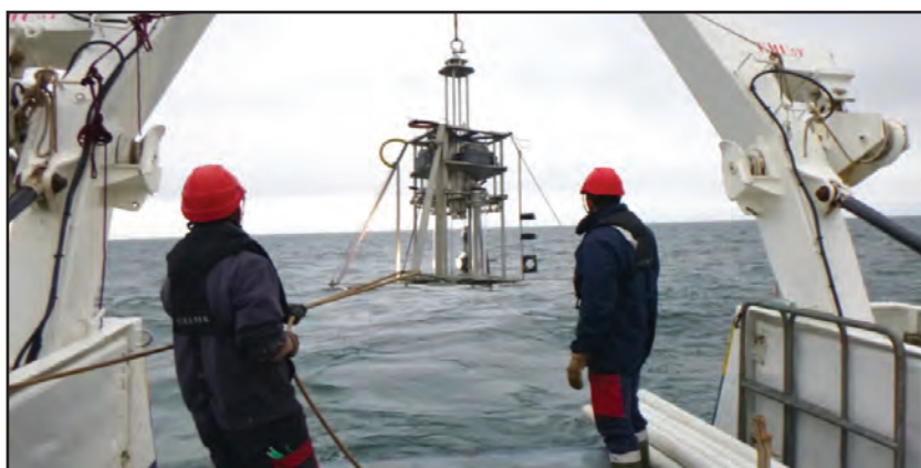
Un carottier multitube utilisé pour la première fois sur un navire côtier est plongé sur le site du Pilier en Loire-Atlantique. Crédit : Ifremer
